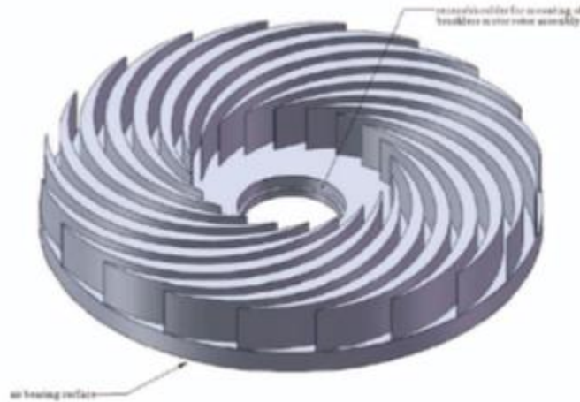
Figure 22. V1 impeller.
